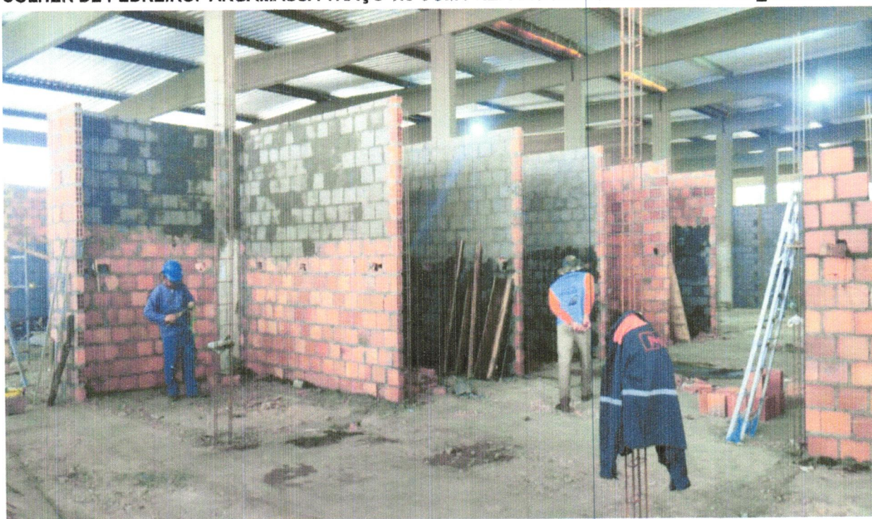
FOTO 34 - CHAPISCO APLICADO EM ALVENARIAS E ESTRUTURAS DE CONCRETO INTERNAS, COM COLHER DE PEDREIRO. ARGAMASSA TRAÇO 1:3 COM PREPARO EM BETONEIRA 400L. AF_10/2022.
