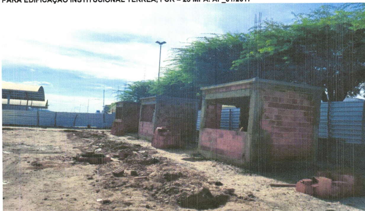
FOTO 58 - (COMPOSIÇÃO REPRESENTATIVA) EXECUÇÃO DE ESTRUTURAS DE CONCRETO ARMADO, PARA EDIFICAÇÃO INSTITUCIONAL TÉRREA, FCK = 25 MPA. AF_01/2017
